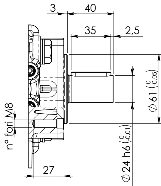
Detailed shaft view Vista dettagliata albero
